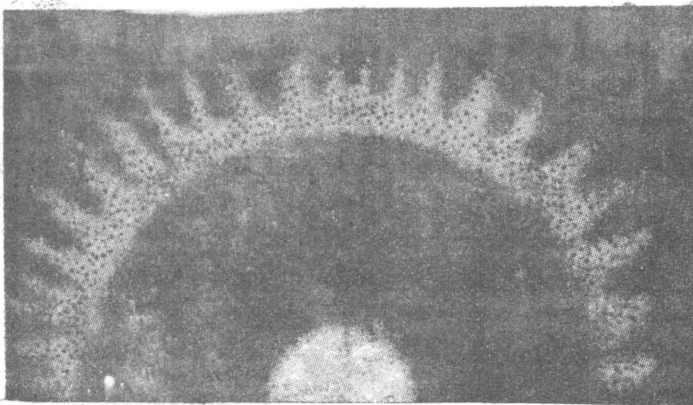
Planetbildningens första skede enligt Fred Hoyle. En gasring har avskiljts från en sol. Ur denna ring kondenseras järn och sten ut och stannar kvar i kretslopp kring solen medan ringen under sin fortsatta utvidgning sveper med sig finare stoftpartiklar till solsystemets yttre regioner. De planeter som ligger nära sin sol – som vår jord – får därmed mycket större täthet än planeterna längre bort.
